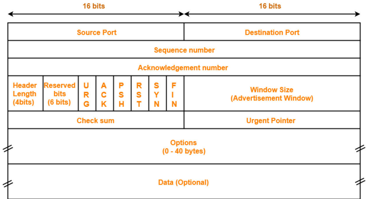
TCP Header
